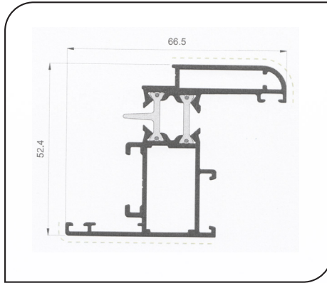
TS 0004 - ARO MÓVEL PEQUENO
