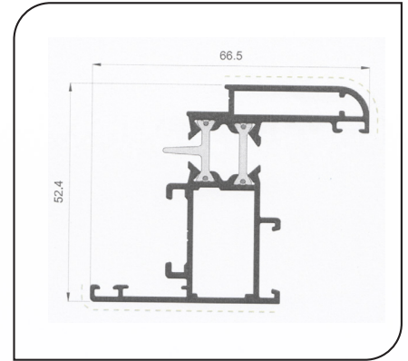
TS 0006 - ARO MÓVEL GRANDE
