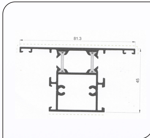
TS 0009 - TRAVESSA PEQUENA
