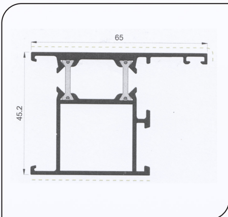
TS 0013 - ARO FIXO GRANDE
