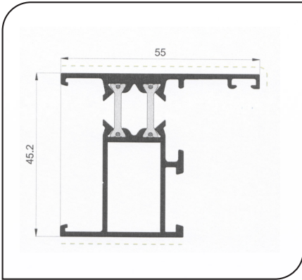
TS 0001 - ARO FIXO
