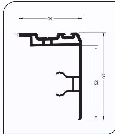
BATENTE 1575506
