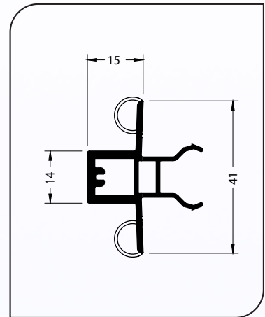
BATENTE 1575507
